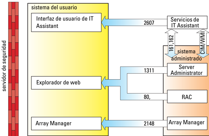
Ilustración 11-1. Instalación típica detrás de un servidor de seguridad
