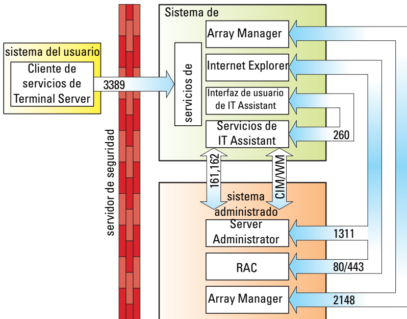
Ilustración 11-2. Cómo utilizar los servicios de Terminal Server para obtener seguridad adicional
